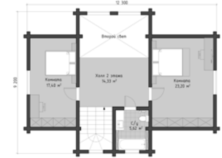
2 этаж
